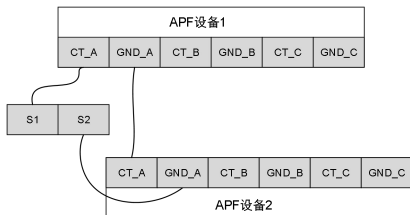
图 3-4 并机时的 CT 串联接法
