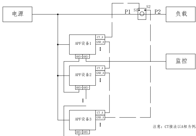
图 3-3 并机时配电与监控接线示意图
