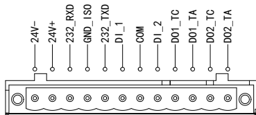
图 2-5 信号端口配置图
