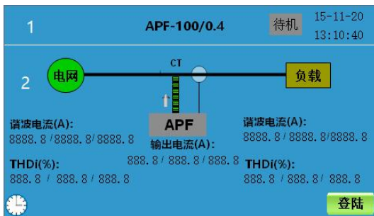
图 4-1 LCD 触摸屏显示主页
