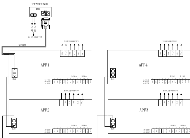
图 3-5 并机时的模块通讯接法
