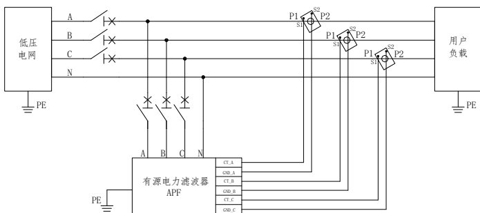
图 3-2 单机配电接线示意图
