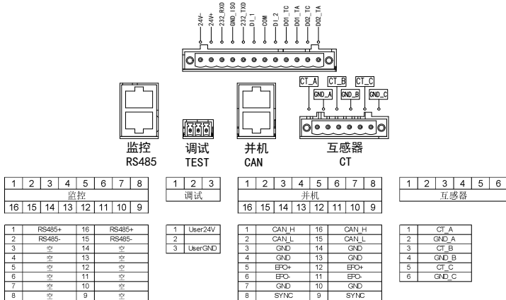
图 2-4 信号端口配置图
